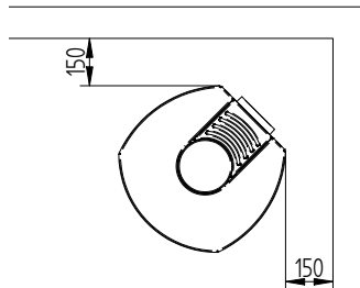
Distance des matériaux inflammables avec conduit de fumée non isolé
