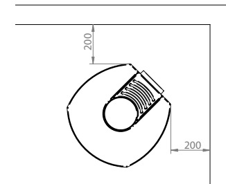
Abstand zu brennbarem Material ohne isoliertem Rauchrohr
