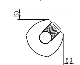
Uten isolerte røykrør
