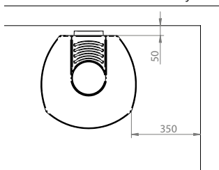
Avstand til brennbart med isolerte røykrør
