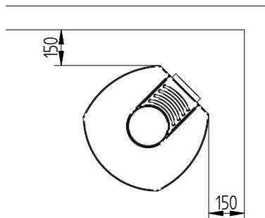
Uden isoleret røgrør
