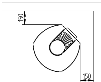
Distanza da materiali infiammabili senza canna fumaria isolata
