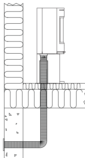
Figur 2C, via de vloer en kelder
