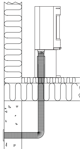
Figur 2C, par le sol et la cave
