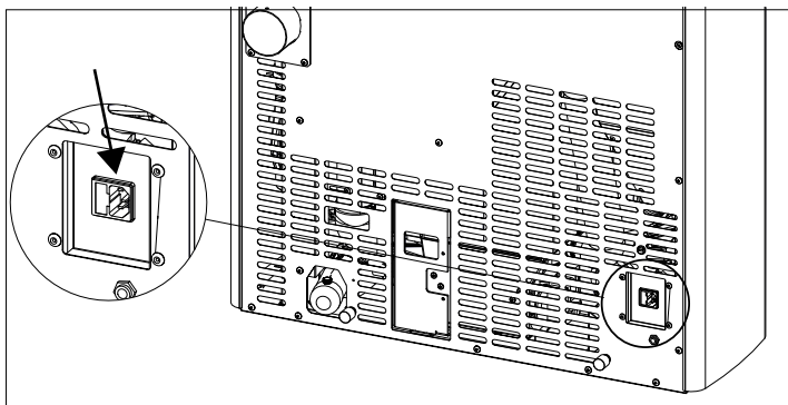
ELEKTRISCHE AANSLUITING VAN DE KACHEL
