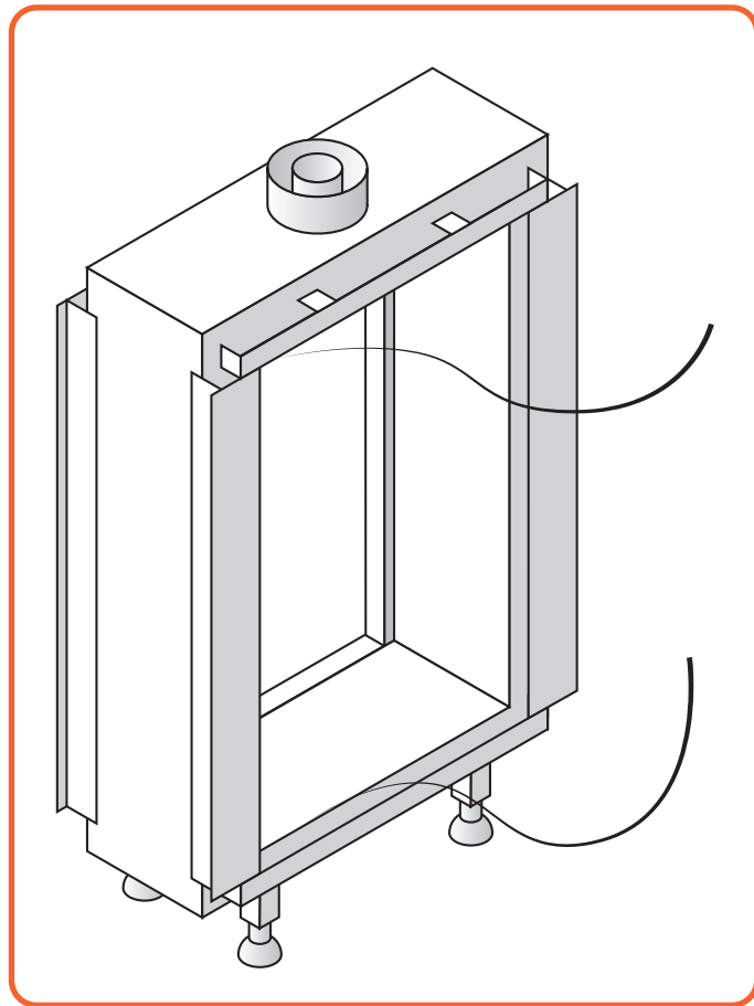
Afb. 10.7 Verwijder glastouw
