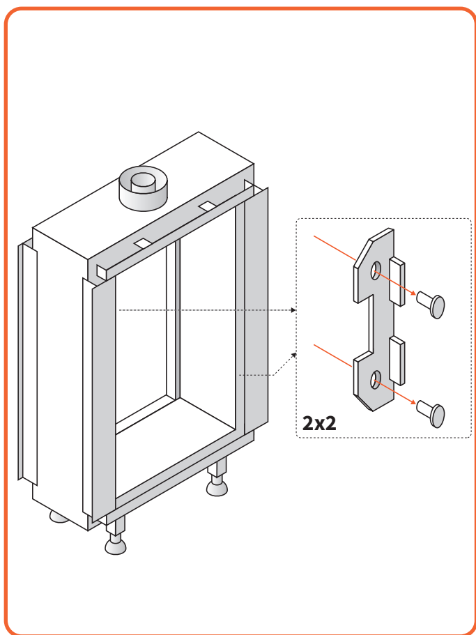
Afb. 10.6 Verwijder glasbeugels
