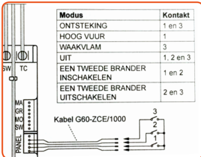
Afbeelding A-14: Domotica systeem
