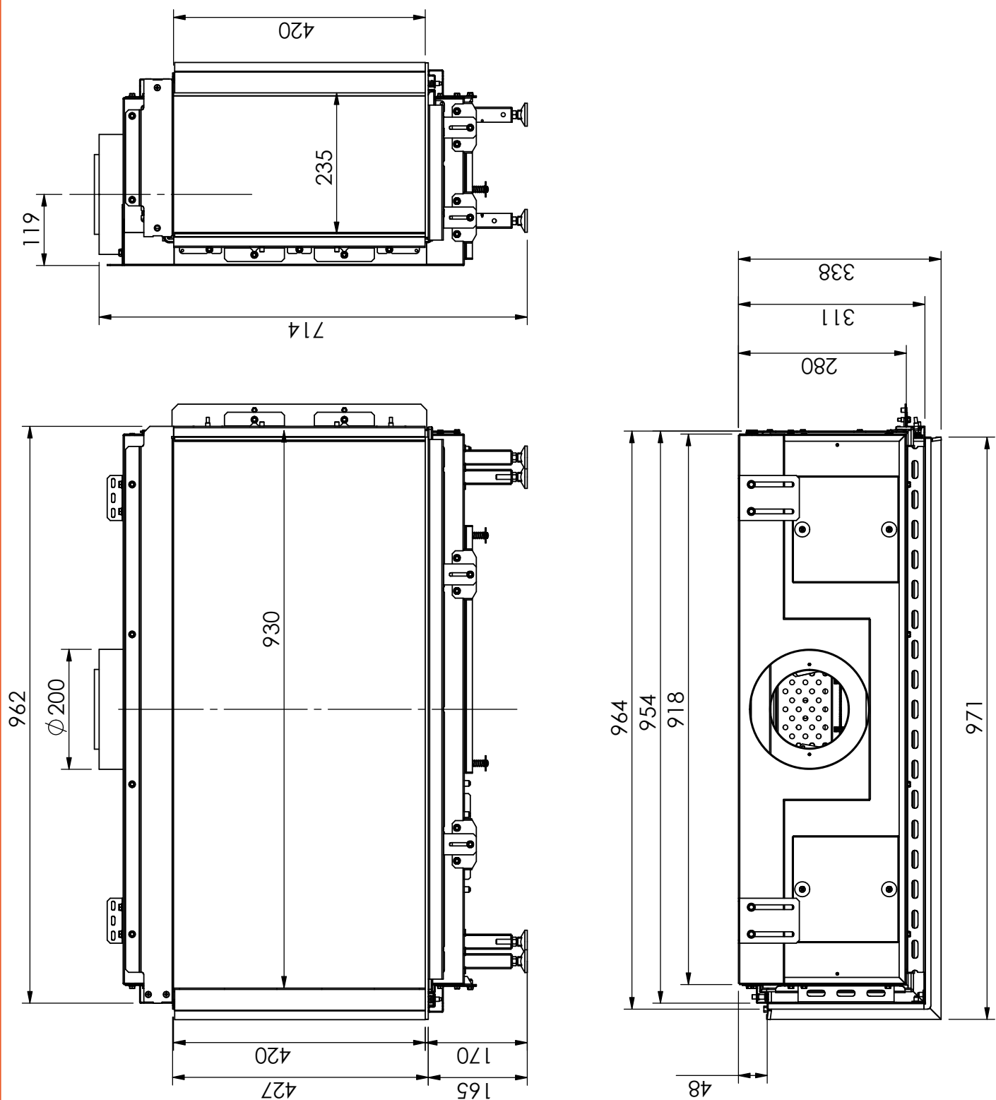
Afbeelding I-3: Lijntekening Bidore100
