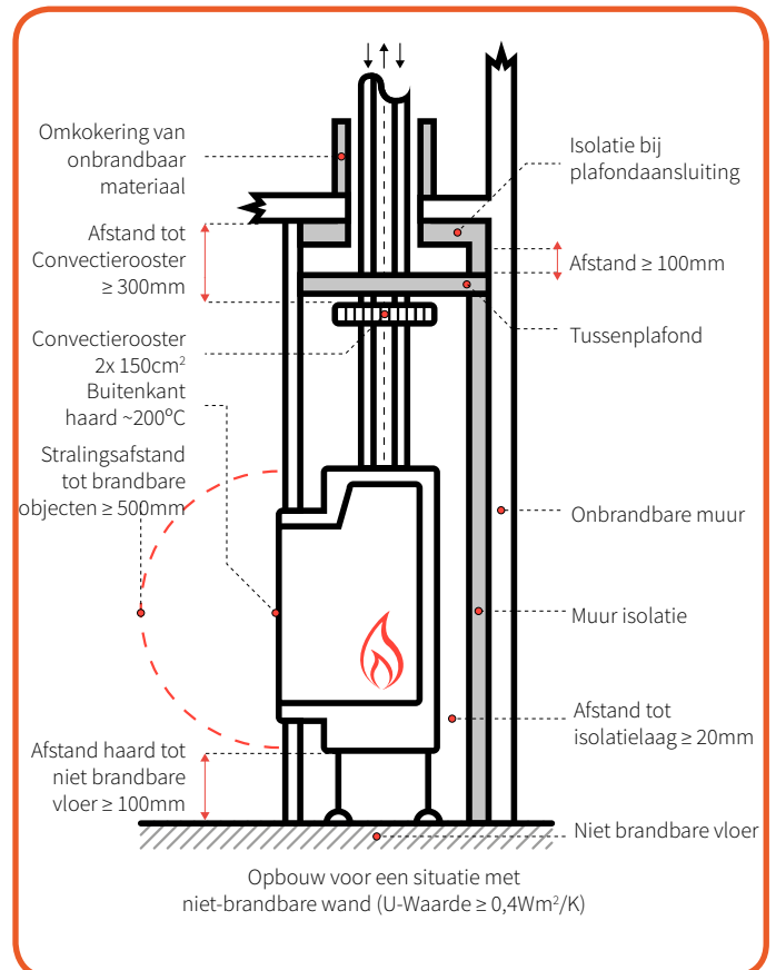
Afb. 6-1: Niet-brandbare wand-/dakmateriaal
