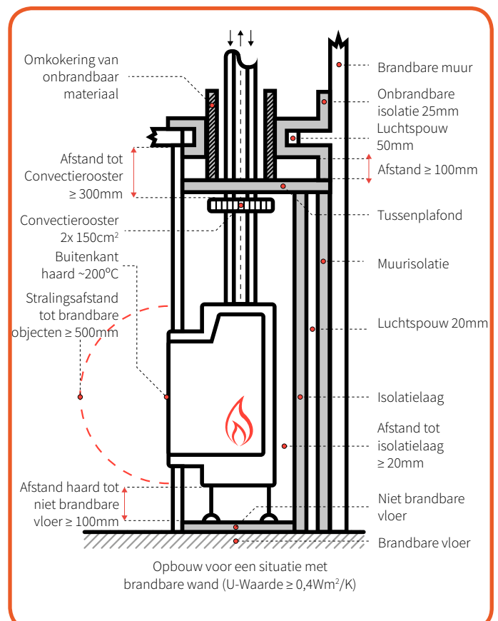
Afb. 6-2: Brandbaar wand-/dakmateriaal bij dakdoorvoer
