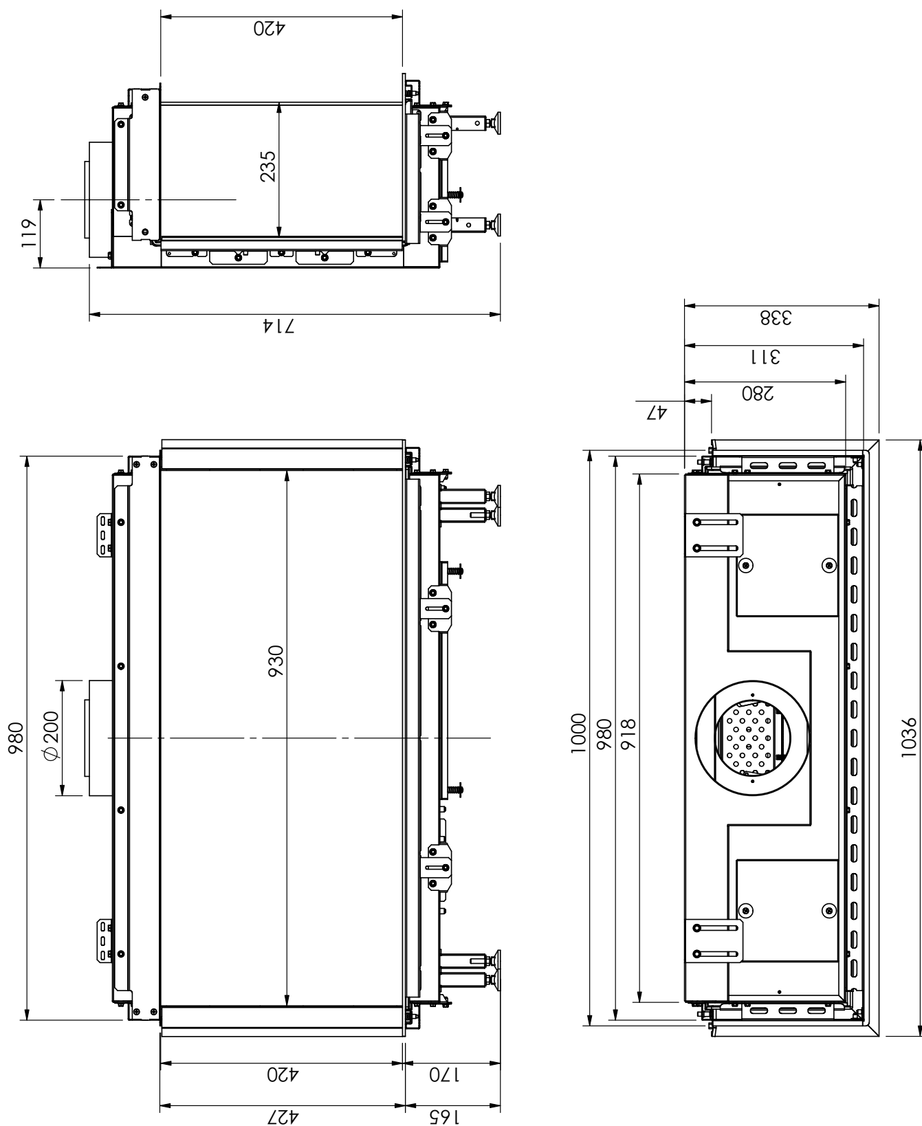
Afbeelding I-4: Lijntekening Trisore100
