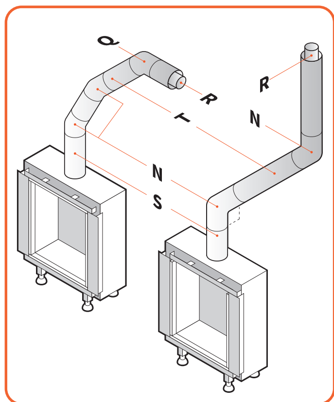
Afb. 7.1 Voorbeelden afvoer
