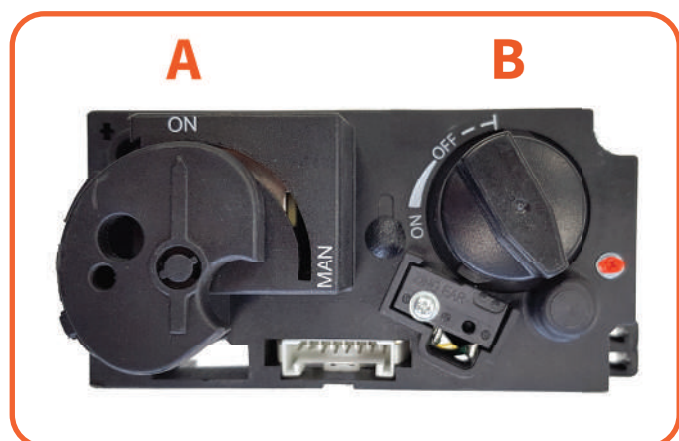
Afb. 4.2 Gasblok; hoofdbrander ontsteking
