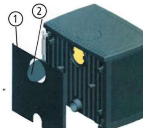
Afbeelding 4.1 Achterwand demonteren
