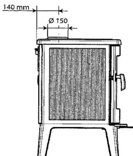
Sortie dessus
