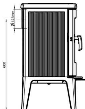
Achteraansluiting
