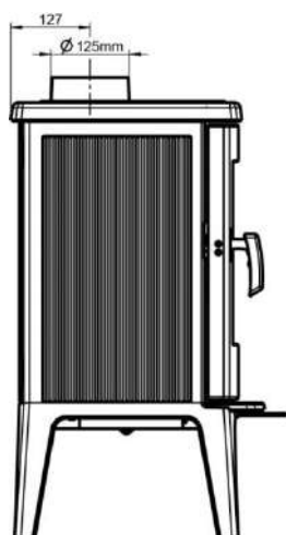
Bovenaansluiting
