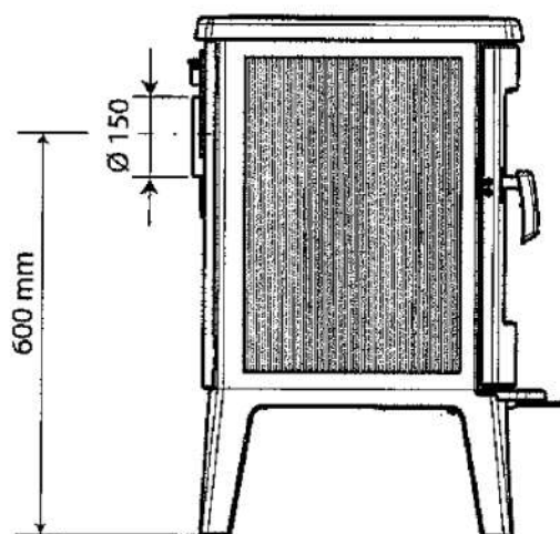
Sortie arrière
