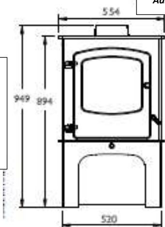
Sokkel met houtvak
