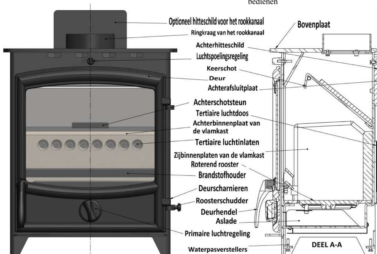
Afb 2 – Montage en bedieningselementen van de FX FP FQ FT Eco. 5 breed-model wordt weergegeven.
