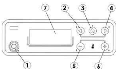
Fig. 7 - Bedieningspaneel
