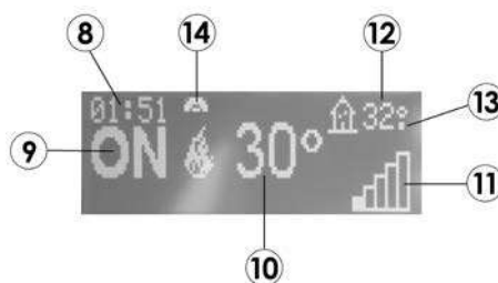
Fig. 10 - Display
