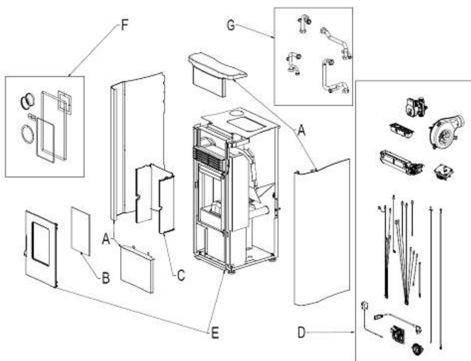
Fig. 1 - Geëxplodeerde tekening
