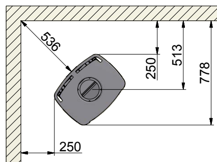
65-2, 65-4, 65-6, 65-8 en 65-10 (met zijglas) Installatie in een hoek van 45°
