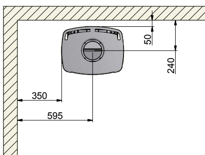
65-1, 65-3, 65-5, 65-7 en 65-9 (zonder zijglas) Parallele installatie
