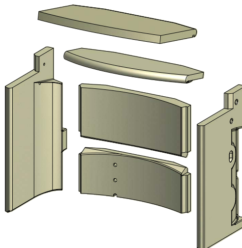
65-1, 65-3, 65-5, 65-7 en 65-9 (zonder zijglas)
