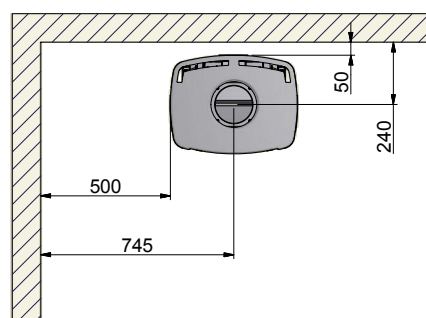
65-2, 65-4, 65-6, 65-8 en 65-10 (met zijglas) Parallele installatie
