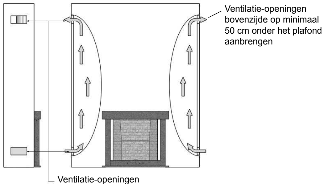
Figuur 2: Toepassing ventilatie schouw
