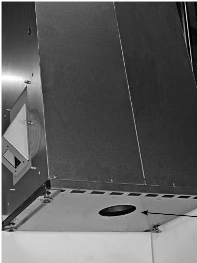
Luchttoevoer-aansluiting onderzijde toestel
