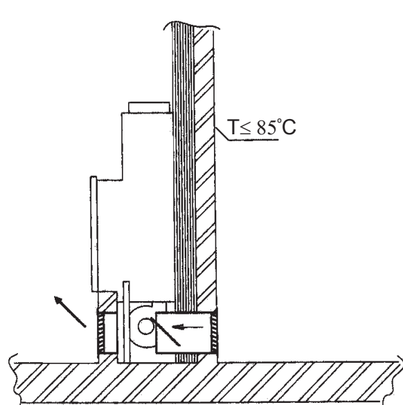
Haard tegen een niet-dragende en onbrandbare wand
