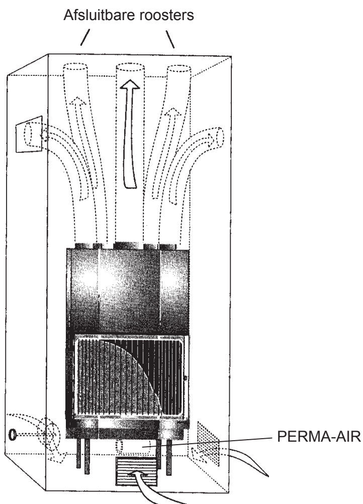
Haard tegen een dragende muur of tegen een wand van brandbare bouwmaterialen
