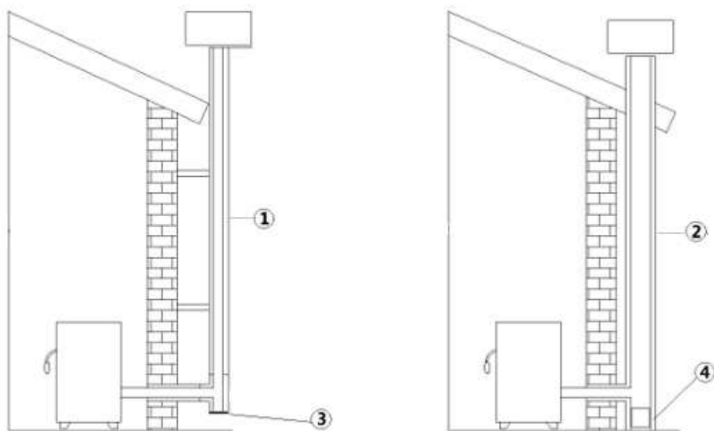
Fig. 3 - Rookkanalen
