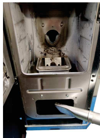
Fig. 80 - Zuig de as op
