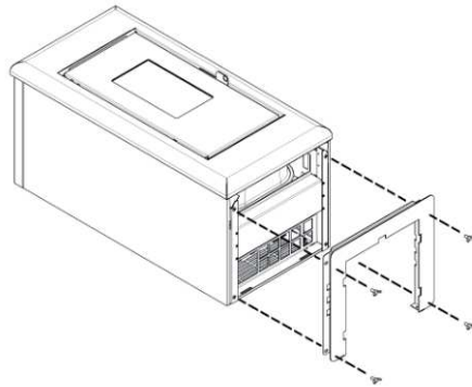
Fig. 50 - Montage sokkel
