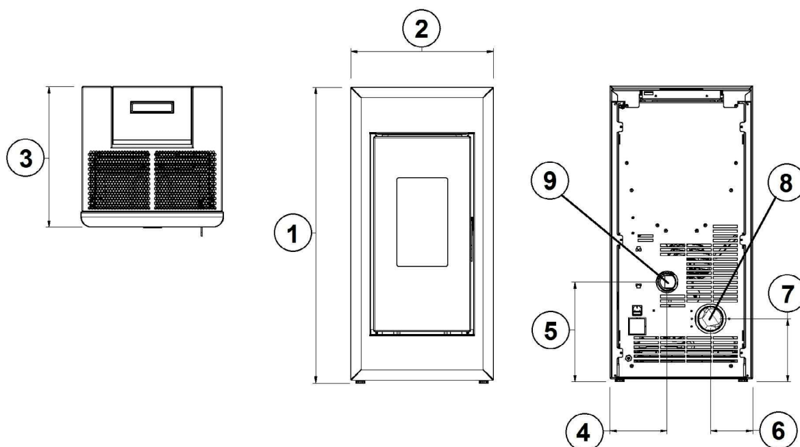
Fig. 20 - Algemene afmetingen: ONE7 - BEAM 7 - ACCENT K7
