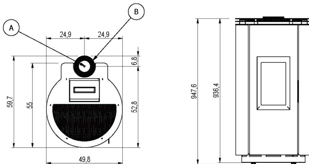
Fig. 19 - Algemene afmetingen: FLOYD 5 - 7 - LORD 7
