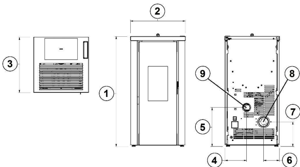
Fig. 23 - Algemene afmetingen: VERA 7
