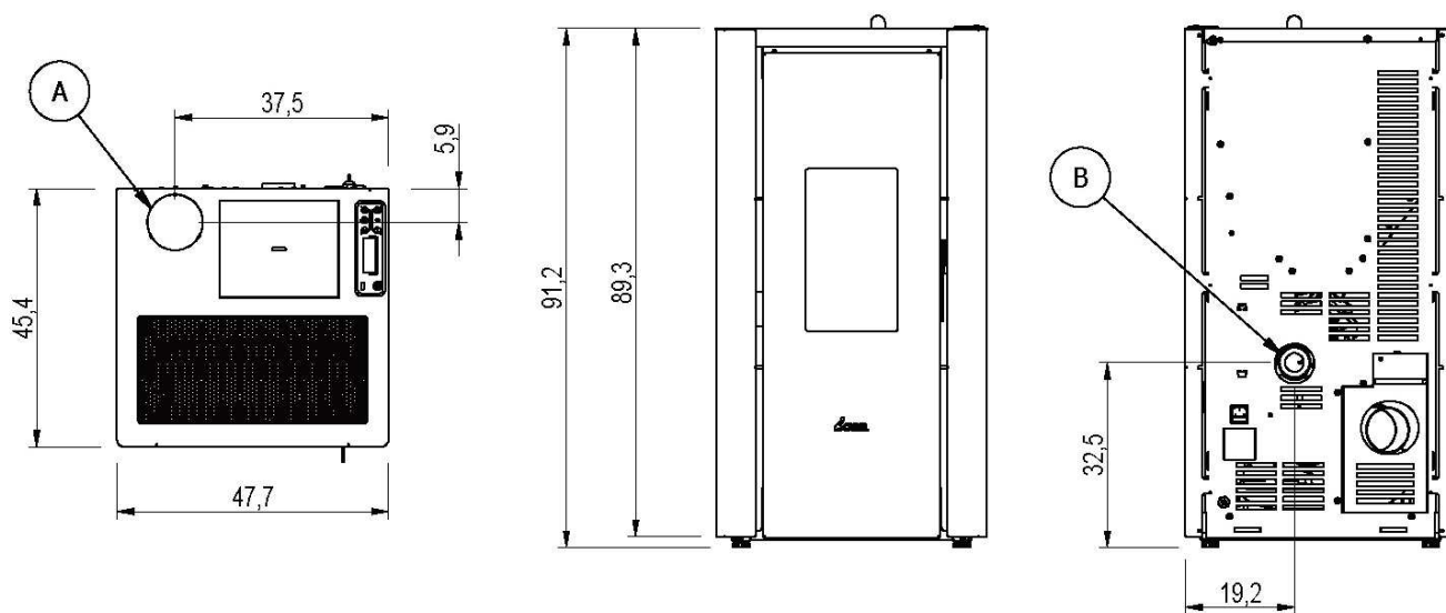
Fig. 26 - Algemene afmetingen: CRISTAL 7 UP
