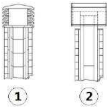
Fig. 5 - Windbestendige schoorsteenpotten
