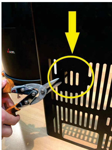
Fig. 61 - Ring breken
