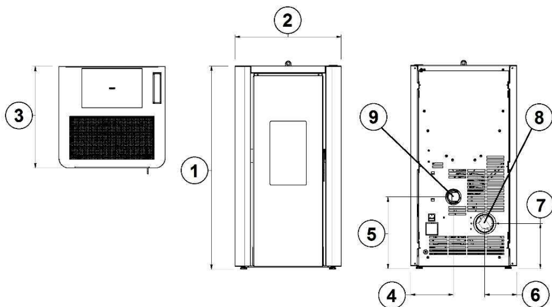
Fig. 24 - Algemene afmetingen: INDIGO 7
