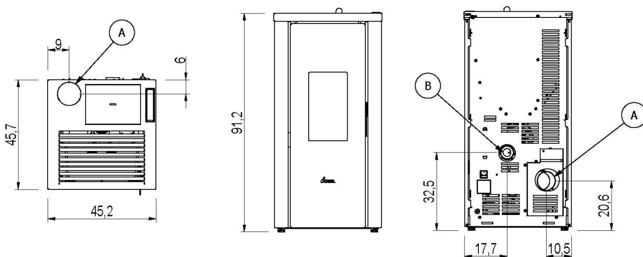
Fig. 25 - Algemene afmetingen: VERA 7 UP
