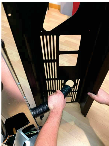
Fig. 64 - Doorgang flexibele buis 2
