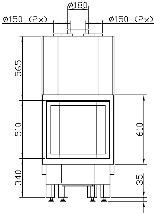
Vooranzicht Frontansicht Vue de face Front view
