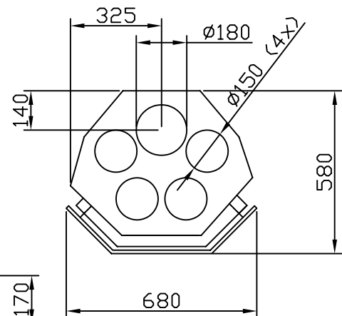
Bovenaanzicht Draufsicht Echangeur Top view
