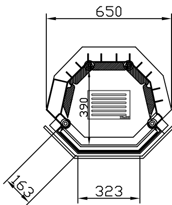
Doorsnede verbrandingskamer Grundriss Feuerstelle Coupe sur foyer Cross section
