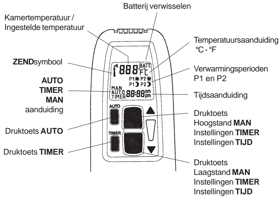
Figuur 4: Handzender
