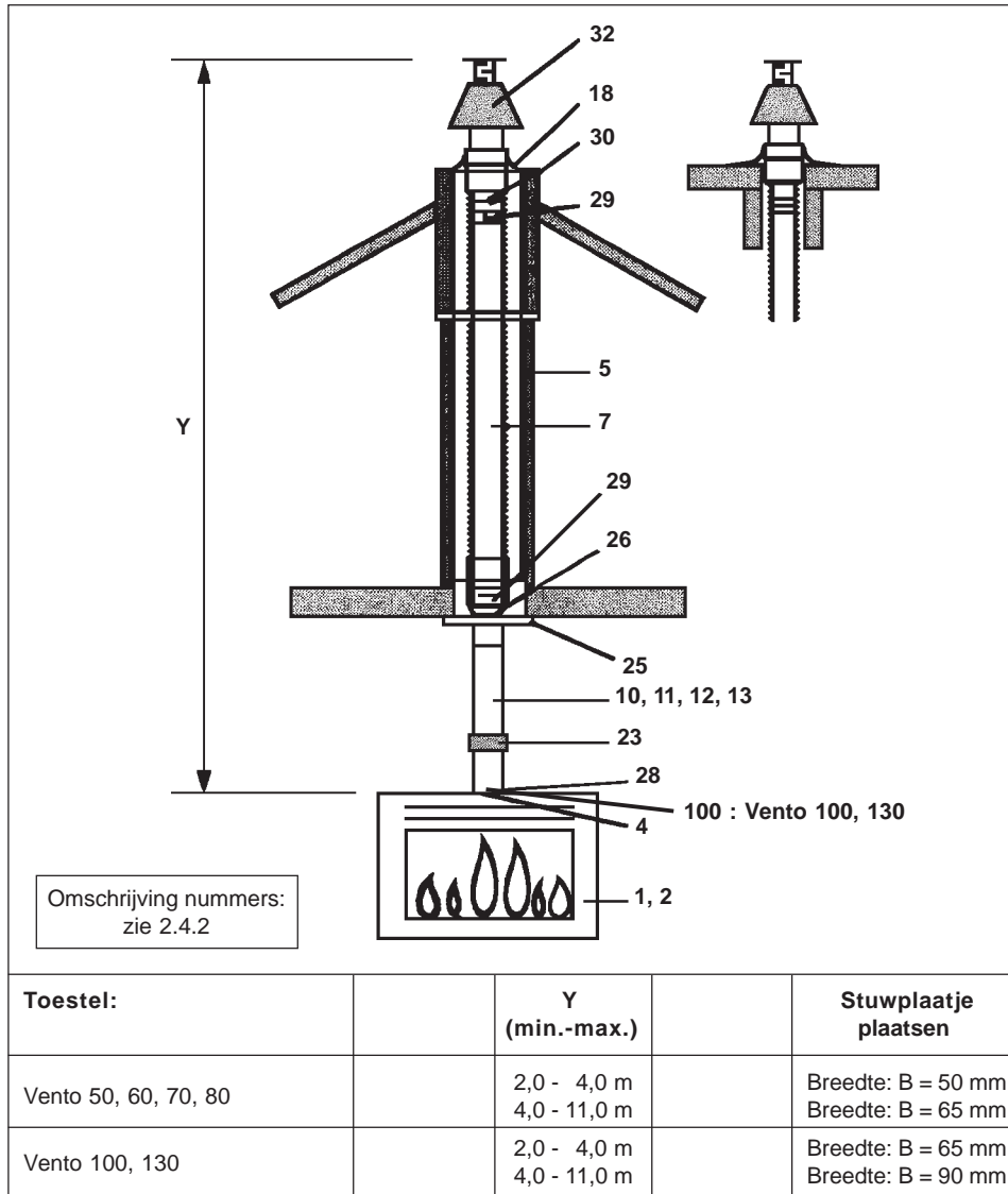
Figuur 16: Verticale schoorsteenuitmondning bij gebruik van een bestaand rookkanaal (Flexibel Ø100 mm en/of star Ø100 mm / Ø150 mm)
